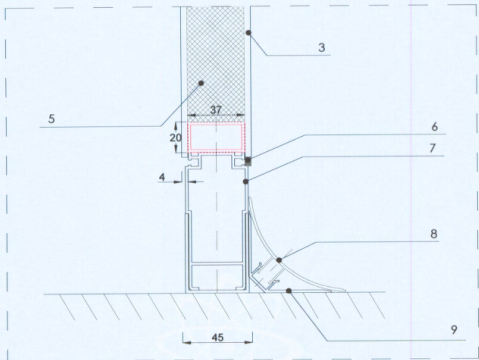
Particolare nodo inferiore.
