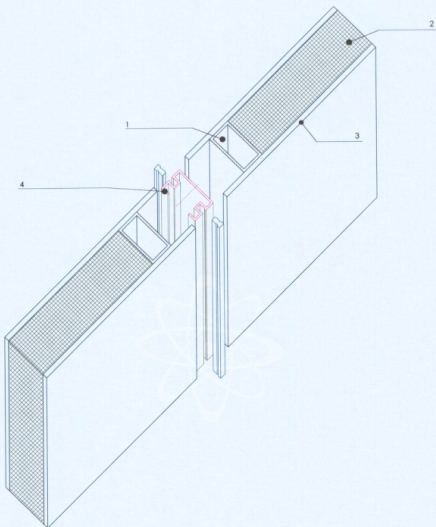
Particolare di assemblaggio nodo centrale.
