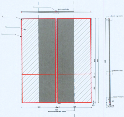
Prospetto della struttura, sezione verticale e orizzontale.
